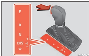
Abb. 85 Wählhebelsperre.
