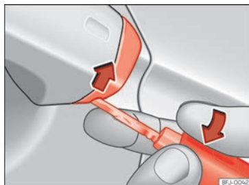
Abb. 52 Fahrtürgriff: Abdeckkappe abhebeln.
