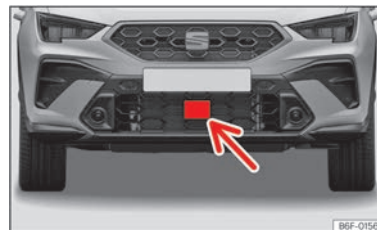
Abb. 92 Im vorderen Stoßfänger: Radarsensor.
