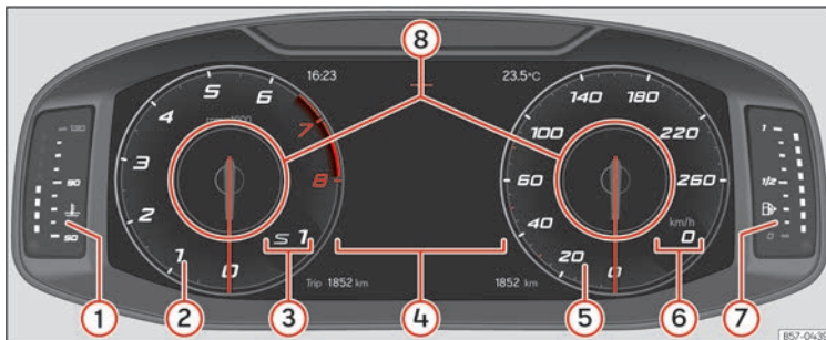
Abb. 2 SEAT Digital Cockpit in der Schalttafel (klassische Ansicht).
