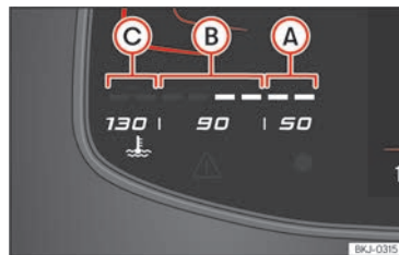
Abb. 5 Digitales Kombi-Instrument Basic: Motorkühlmitteltemperatur-Anzeige.
