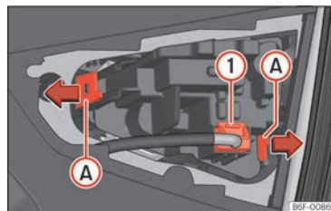
Abb. 173 Lampenträger ausbauen.
