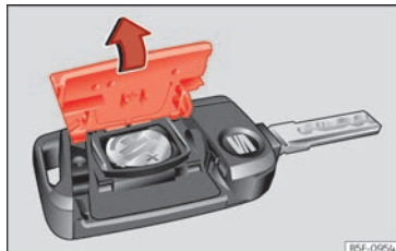
Abb. 45 Fahrzeugschlüssel: Deckel des Batteriefachs öffnen.
