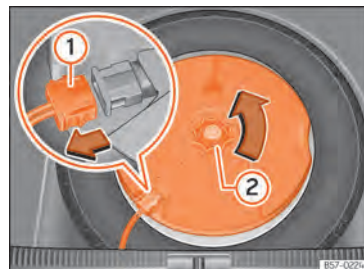
Abb. 221 Im Gepäckraum: Subwoofer ausbauen.
