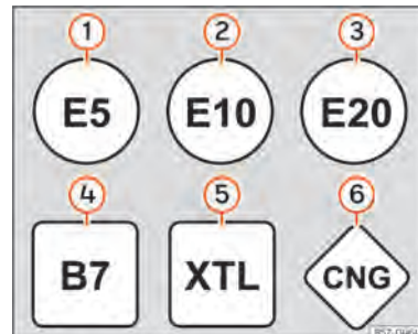
Abb. 187 Kraftstoffkennzeichnung nach EU-Richtlinie 2014/94/EU.
