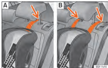
Abb. 39 Rücksitze: Einstellung und Einbau unter Verwendung des Top Tether-Gurts.
