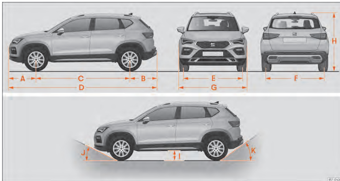
Abb. 234 Abmessungen
