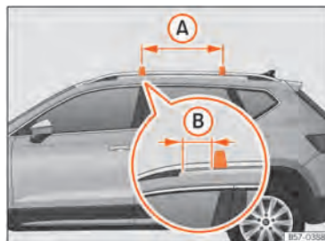
Abb. 180 Befestigungspunkte der Querstangen für den Dachgepäckträger.
