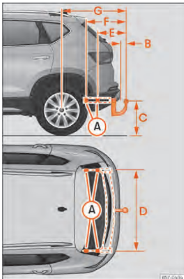
Abb. 185 Maße und Befestigungspunkte für den nachträglichen Einbau einer Anhängervorrichtung
