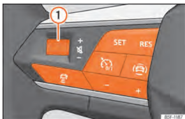
Abb. 66 Bedienelemente am Lenkrad
