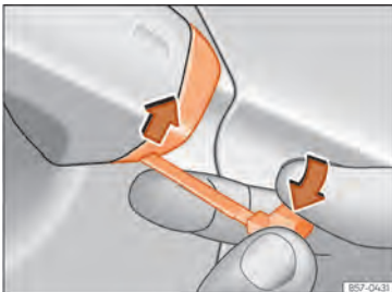
Abb. 53 Fahrertürgriff: Abdeckkappe abhebeln.
