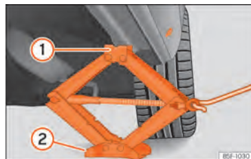
Abb. 227 Längsträger: Wagenheber ansetzen.
