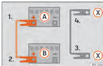
Abb. 194 Anschlussplan für Fahrzeuge mit Start-Stopp-System.
