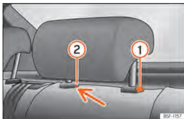
Abb. 75 Kopfstütze hinten ausbauen.
