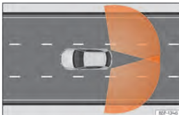
Abb. 109 Erfassungsbereich der Sensoren.
