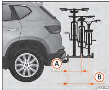
Abb. 184 Schematische Darstellung des maximalen Überstands der Ladung in einem Fahrradträger für zwei oder drei Fahrräder.
