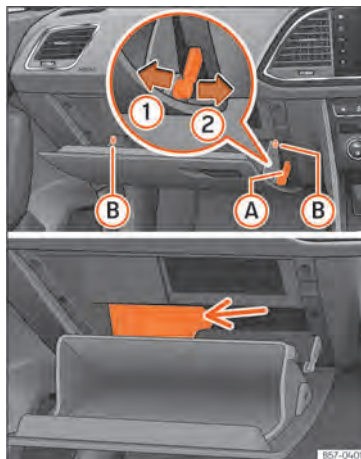
Abb. 201 Rechtslenker: Abdeckung des Sicherungskastens an der Instrumententafel, Beifahrerseite.
