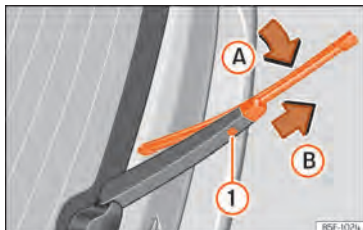
Abb. 192 Scheibenwischerblatt der Heckscheibe auswechseln.
