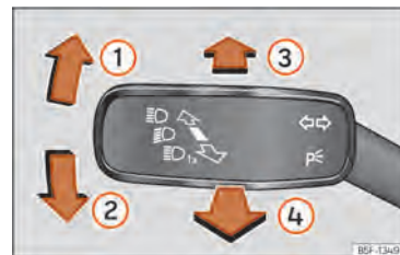
Abb. 81 Blinker- und Fernlichthebel.
