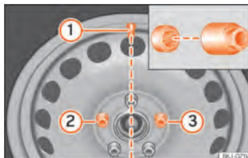
Abb. 225 Radwechsel: Reifenventil ① und Einbauort der Anti-Diebstahl-Radschraube ② oder ③.
