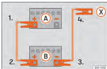
Abb. 193 Anschlussplan für Fahrzeuge ohne Start-Stopp-System.
