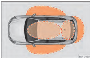
Abb. 48 Keyless-Access: Näherungsbereiche.
