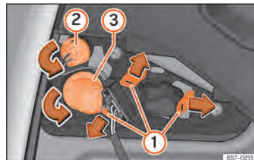
Abb. 205 Lampenträger ausbauen.
