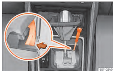
Abb. 101 Wählhebel: Notentriegelung aus der Parkstellung
