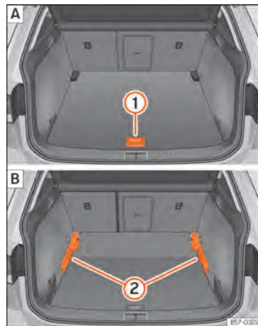
Abb. 171 Variabler Gepäckraumboden: A Hochstellung; B Tiefstellung.
