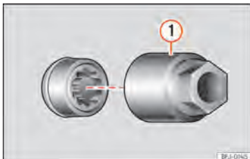
Abb. 223 Diebstahlhemmende Radschraube mit Abdeckkappe und Adapter.
