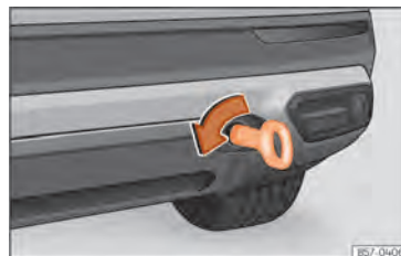
Abb. 199 Auf der rechten Seite des hinteren Stoßfängers: Eingeschraubte Abschleppöse.
