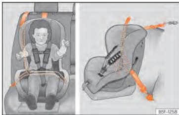
Abb. 40 Auf den Rücksitzen: Einbau von Kindersitzen.
