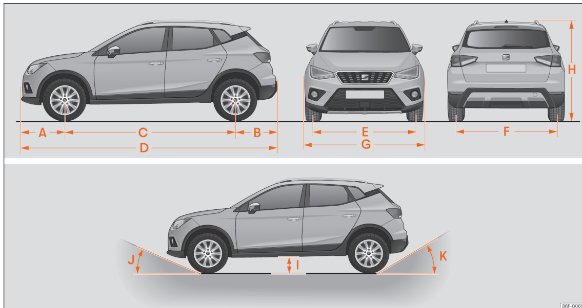
Abb. 293 Abmessungen und Winkel.
