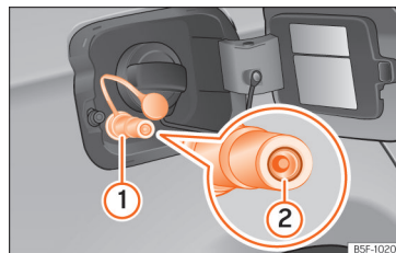
Abb. 274 Geöffnete Tankklappe: Gas-Einfüllstutzen (1), Dichtungsring des Einfüllstutzens (2).
