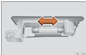
Abb. 66 Gepäckraumleuchte*
