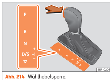
Abb. 214 Wählhebelsperre.
