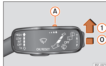
Abb. 113 Scheibenwischerhebel: Regensensor einstellen (A).
