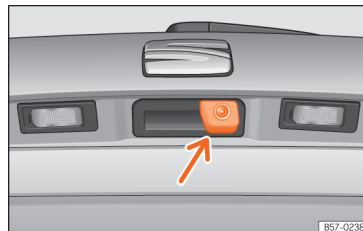
Abb. 260 Im Griff der Heckklappe: Einbauort der Kamera des Rückfahrassistenten.
