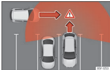
Abb. 124 Schematische Abbildung des Ausparkassistenten: Überwachter Bereich des ausparkenden Fahrzeugs.
