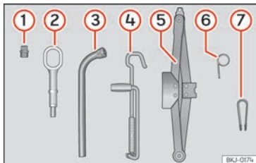
Abb. 148 Im Gepäckraum unter der Ladebodenabdeckung: Bordwerkzeug.
