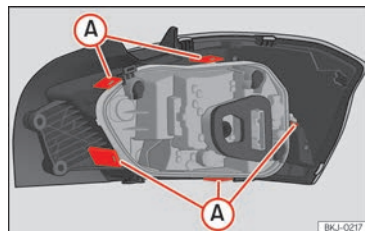
Abb. 163 Befestigungsglaschen Rückseite Heckleuchte.
