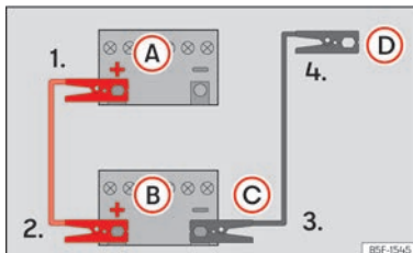
Abb. 152 Anschlussplan für Fahrzeuge ohne Start-Stopp-System.
