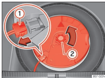
Abb. 181 Im Gepäckraum: Subwoofer ausbauen.
