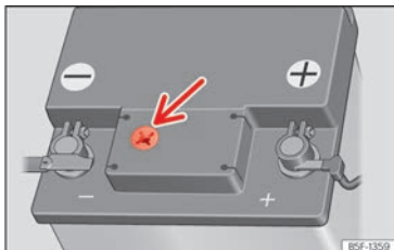
Abb. 177 Sichtfenster an der Oberseite der 12-Volt-Fahrzeugbatterie (Prinzipdarstellung).
