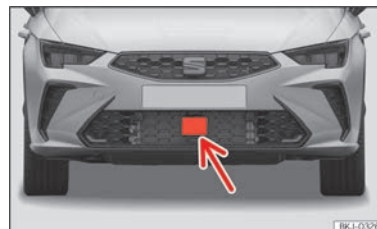
Abb. 94 Im vorderen Stoßfänger: Radarsensor.
