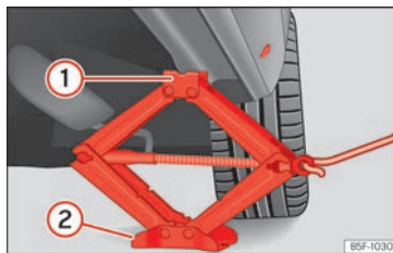
Abb. 189 Längsträger: Wagenheber ansetzen.
