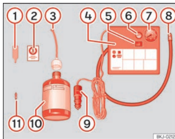
Abb. 191 Prinzipdarstellung: Bestandteile des Pannensets.
