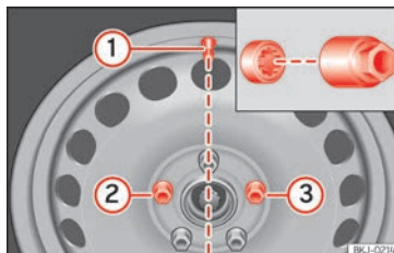
Abb. 187 Radwechsel: Reifenventil (1) und Einbauort der Anti-Diebstahl-Radschraube (2) oder (3).
