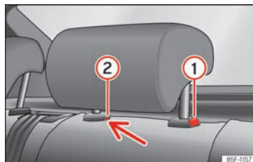
Abb. 68 Kopfstütze hinten ausbauen.
