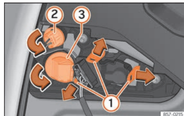
Abb. 206 Lampenhalter ausbauen.
