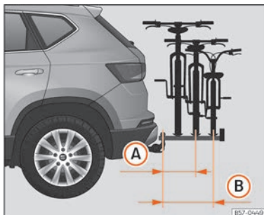
Abb. 186 Schematische Darstellung des maximalen Überstands der Ladung in einem Fahrradträger für zwei oder drei Fahrräder.
