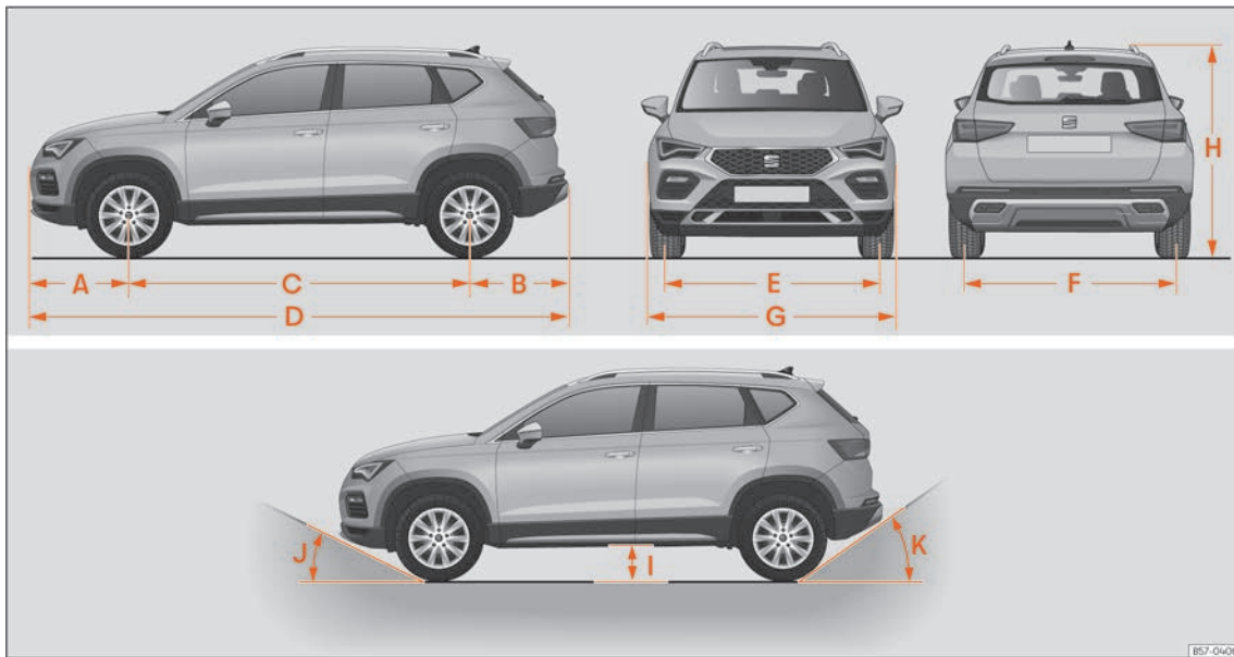
Abb. 235 Abmessungen
