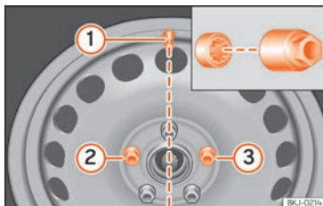
Abb. 227 Radwechsel: Reifenventil ① und Einbauport der Anti-Diebstahl-Radschraube ② oder ③.
