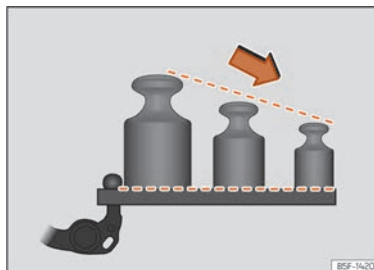
Abb. 185 Empfohlene Gewichtsverteilung im Heckträgersystem.
