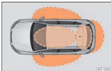
Abb. 51 Keyless-Access: Näherungsbereiche.
