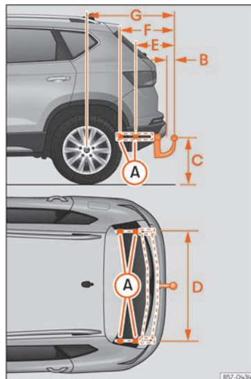
Abb. 187 Maße und Befestigungspunkte für den nachträglichen Einbau einer Anhängervorrichtung
