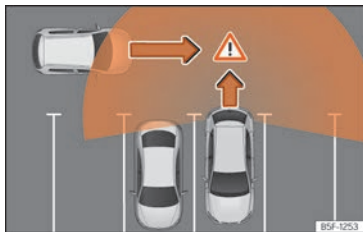
Abb. 154 Schematische Abbildung des Ausparkassistenten: Überwachter Bereich des ausparkenden Fahrzeugs.
