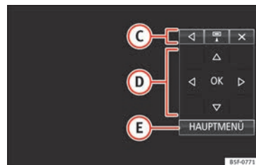
Abb. 26 DVD-Betrieb: Menüsteuerung.
