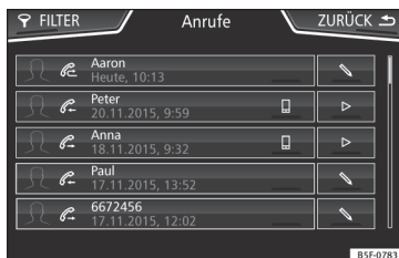
Abb. 57 Menü Anruflisten.
