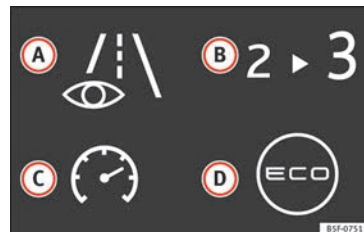
Abb. 47 Fahrstil-Symbole.
