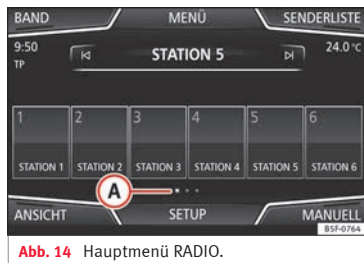
Abb. 14 Hauptmenü RADIO.
