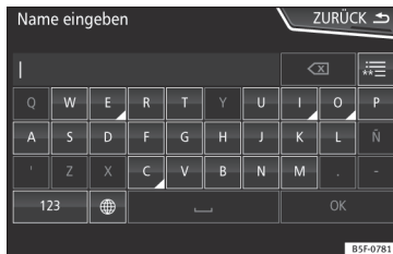
Abb. 55 Suchmaske.
