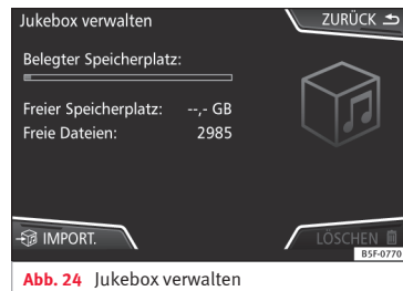
Abb. 24 Jukebox verwalten
