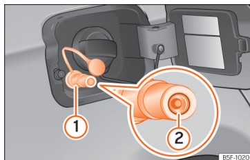
Abb. 156 Geöffnete Tankklappe: Gas-Einfüllstutzen (1), Dichtring des Einfüllstutzens (2).
