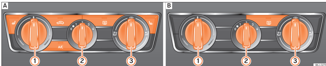
Abb. 82 Auf der Mittelkonsole: A Bedienungselemente der manuellen Klimaanlage; B Bedienungselemente des Heiz- und Frischluftsystems.
