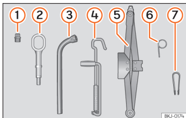
Abb. 158 Im Gepäckraum unter dem Gepäckraumboden: Bordwerkzeug.
