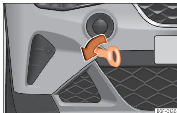
Abb. 165 Vorderer Stoßfänger rechts: Eingeschraubte Abschleppöse
