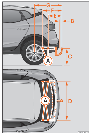
Abb. 152 Maße und Befestigungspunkte für den nachträglichen Einbau einer Anhangervorrichtung
