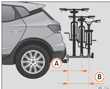
Abb. 151 Schematische Darstellung des maximalen Überstands der Ladung in einem Fahrradträger für zwei oder drei Fahrräder.
