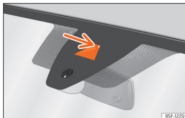
Abb. 97 Kamerasichtfenster des Spurhalteassistenten.
