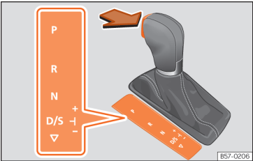
Abb. 88 Wählhebelsperre.
