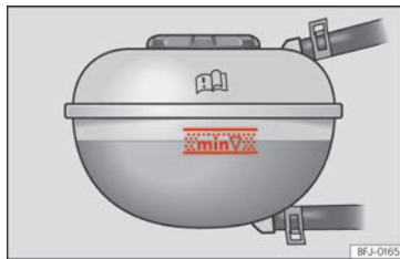
Abb. 208 Im Frontraum: Markierung am Kühlmittelausgleichsbehälter.
