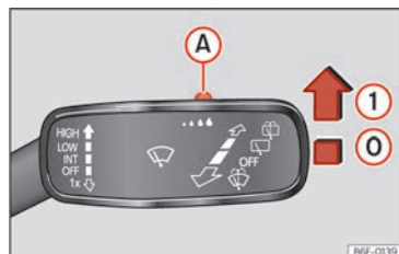
Abb. 84 Scheibenwischerhebel: Regensensor (A) einstellen.
