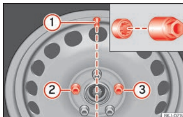
Abb. 225 Radwechsel: Reifenventil ① und Einbaulage der Anti-Diebstahl-Radschraube ② oder ③.
