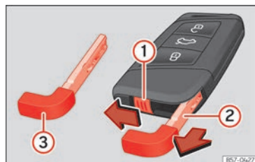
Abb. 45 Fahrzeugschlüssel: Notschlüssel abziehen.
