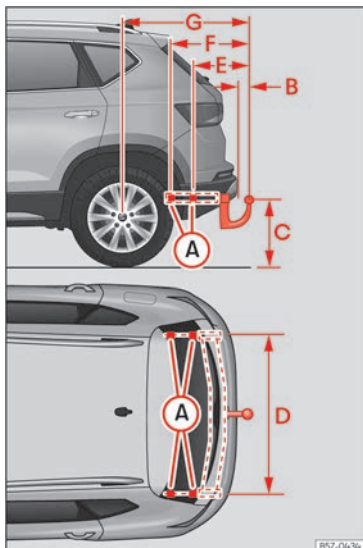
Abb. 185 Anhängervorrichtung: Maße und Befestigungspunkte.
