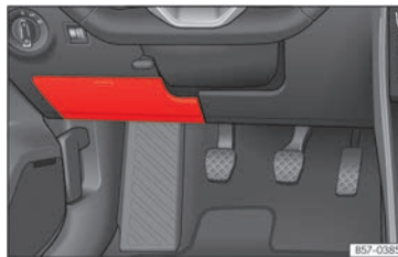
Abb. 200 Auf der Fahrerseite in der Schalttafel: Abdeckung des Sicherungskastens.
