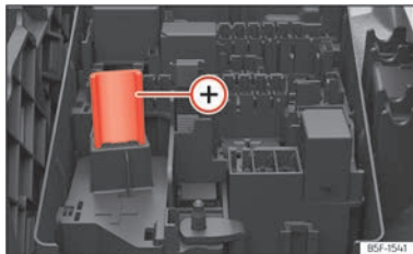
Abb. 216 Im Motorraum unter der Abdeckung des Sicherungskastens: Plus-Anschlusspunkt.
