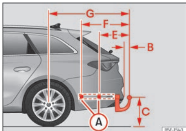
Abb. 207 Anhängervorrichtung: Maße und Befestigungspunkte.
