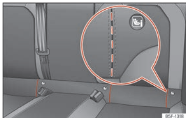
Abb. 40 Rücksitz: eingetragte Schlitz für Zugriff auf die ISOFIX/i-Size-Halteösen.
