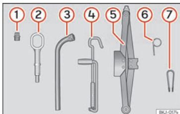
Abb. 213 Im Gepäckraum unter der Ladebodenabdeckung: Bordwerkzeug.
