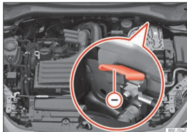
Abb. 217 Im Motorraum, rechts, neben dem Wasserkasten: Minus-Anschlusspunkt.
