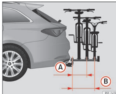
Abb. 206 Schematische Darstellung des maximalen Überstands der Ladung in einem Fahrradträger für zwei oder drei Fahrräder.
