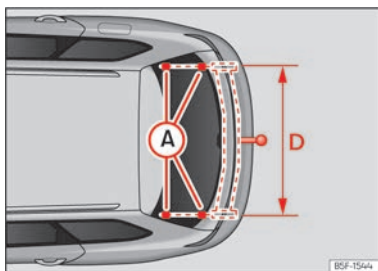
Abb. 208 Anhängervorrichtung: Maße und Befestigungspunkte.
