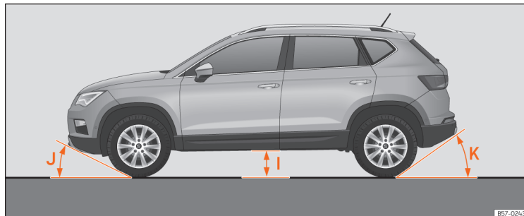
Abb. 314 Abmessungen
