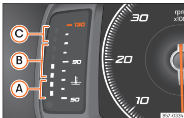
Abb. 131 Frei konfigurierbares Kombi-Instrument: Motorkühlmitteltemperatur-Anzeige.
