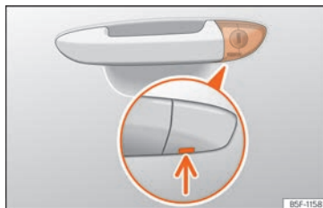
Abb. 53 Fahrtürgriff: verborgener Schließzylinder.
