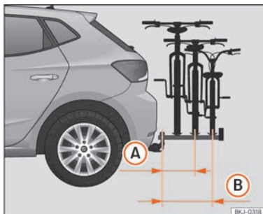
Abb. 147 Schematische Darstellung des maximalen Überstands der Ladung in einem Fahrradträger für zwei oder drei Fahrräder.
