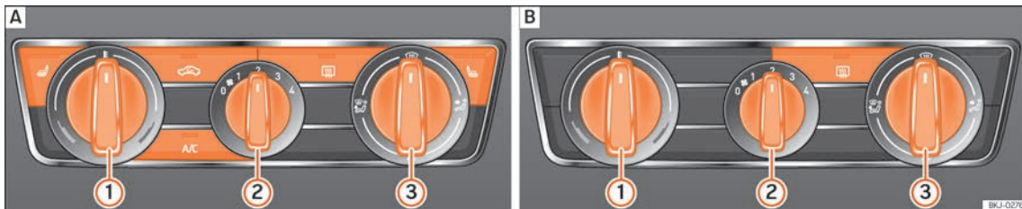
Abb. 83 Auf der Mittelkonsole: A Bedienungselemente der manuellen Klimaanlage; B Bedienungselemente des Heiz- und Frischluftsystems.
