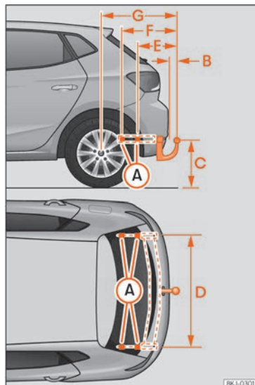
Abb. 148 Maße und Befestigungspunkte für den nachträglichen Einbau einer Anhängervorrichtung
