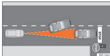
Abb. 111 Abbiegendes und weiteres stehendes Fahrzeug.
