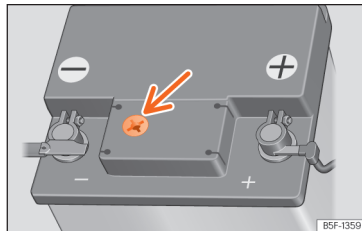
Abb. 230 Sichtfenster an der Oberseite der 12-Volt-Fahrzeuggelbatterie (Prinzipdarstellung).
