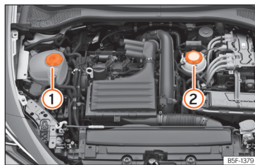
Abb. 220 Motorraum: Kühlmittelbehälter
