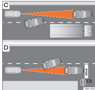
Abb. 135 [C] Fahrspurwechsel eines anderen Fahrzeugs. [D] Abbiegendes und weiteres stehendes Fahrzeug.
