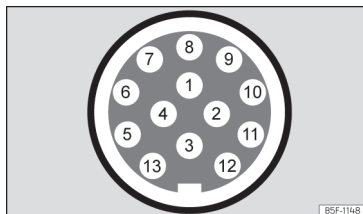
Abb. 197 Schematische Darstellung: Zuweisung der Steckverbinderstifte für Anhängerstrom.
