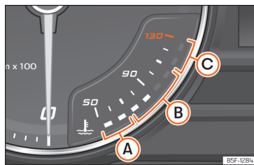
Abb. 9 Analoges Kombi-Instrument: Motorkühlmitteltemperatur-Anzeige.
