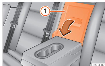
Abb. 193 An der Rücksitzlehne: Öffnung der Durchladeeinrichtung.
