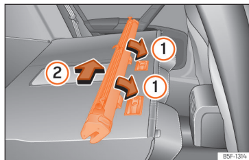
Abb. 186 Einbau des Trennnetzes an den Rücksitzlehnen
