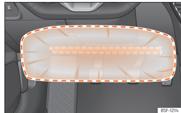
Abb. 40 Auf der Fahrerseite: Wirkungsbereich des Knieairbags.
