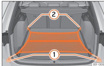
Abb. 189 Im Gepäckraum: flach eingehängtes Gepäckraumnetz.
