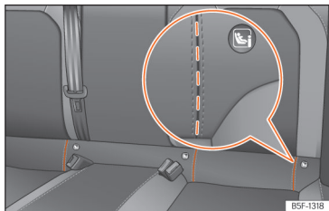
Abb. 44 Rücksitz: eingetragene Schlitze für Zugriff auf die ISOFIX/i-Size-Halteösen.
