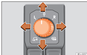
Abb. 109 Ausschnitt der Fahrertür: Außenspiegelbedienung.
