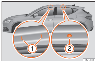
Abb. 196 Befestigungspunkte der Längsträger für den Dachgepäckträger (Leon).
