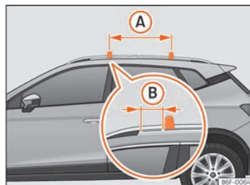
Abb. 150 Befestigungspunkte der Längsträger für den Dachgepäckträger
