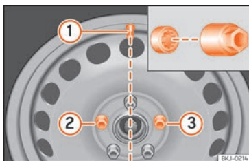
Abb. 198 Radwechsel: Reifenventil ① und Einbaupunkt der Anti-Diebstahl-Radschraube ② oder ③.
