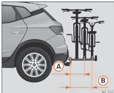
Abb. 153 Schematische Darstellung des maximalen Überstands der Ladung in einem Fahrradträger für zwei oder drei Fahrräder.
