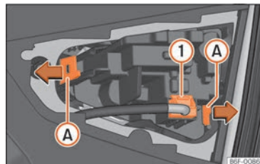
Abb. 175 Lampenhalter ausbauen.
