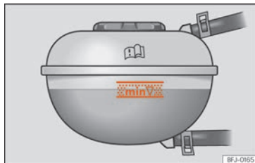
Abb. 181 Im Frontraum: Markierung am Kühlmittelausgleichsbehälter.
