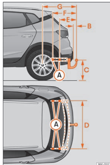
Abb. 154 Maße und Befestigungspunkte für den nachträglichen Einbau einer Anhangervorrichtung
